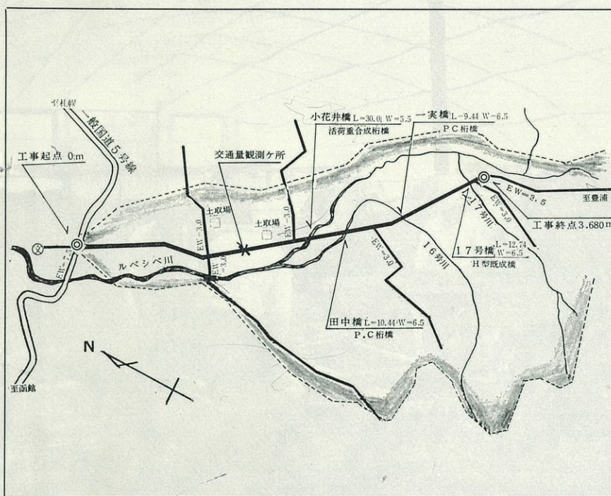
〔工事の完成略図〕
