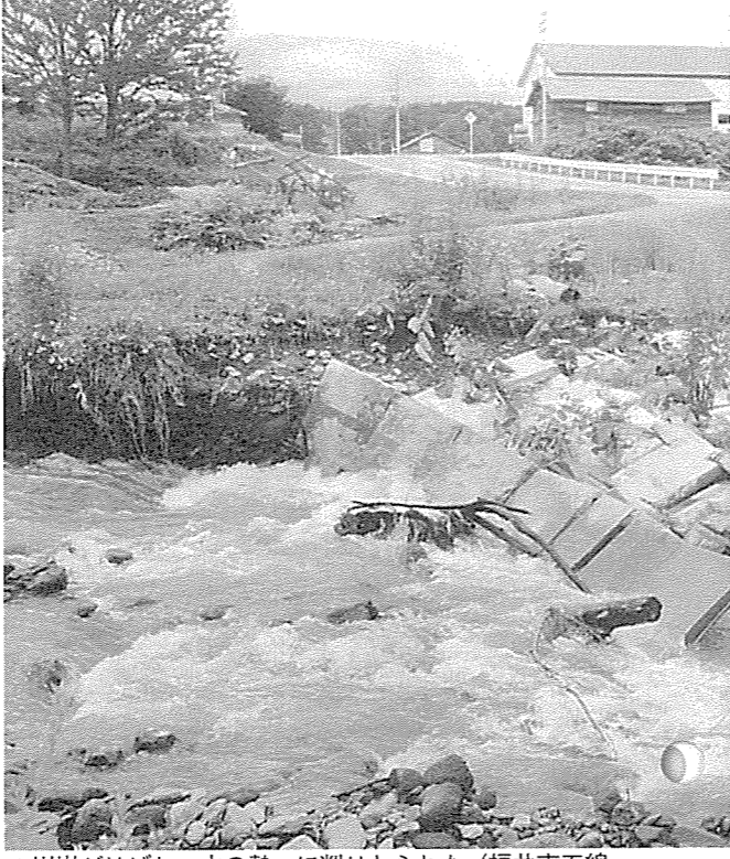
▲川岸がはげしい水の勢いに削りとられた(福井南五線、名無川にかかる入倉橋下の護岸)
