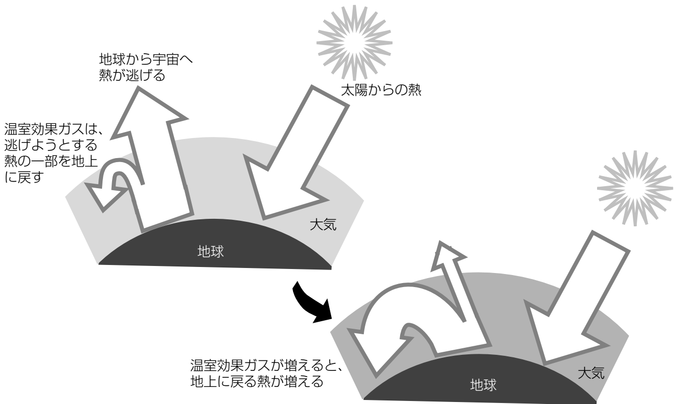
図1 地球温暖化のメカニズム
