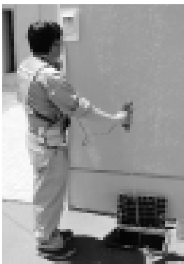
写真1 地下に埋設された水道メーターに伝わる小さな振動音を探り当て、漏水の有無を調査します
